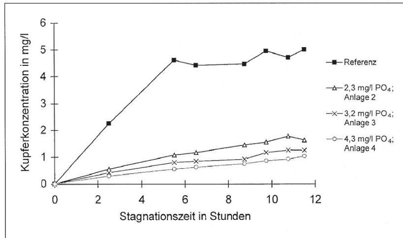
Abb. 1: Kupferkonzentration des Wassers in Abhängigkeit von der Stagnationszeit in Kupferrohren; Alter der Deckschicht: 200 Tage (2)
