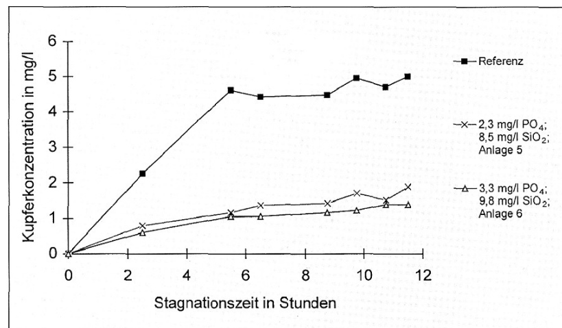
Abb. 2: Kupferkonzentration des Wassers in Abhängigkeit der Stagnationszeit in Kupferrohren; Alter der Deckschicht: 200 Tage (2)
