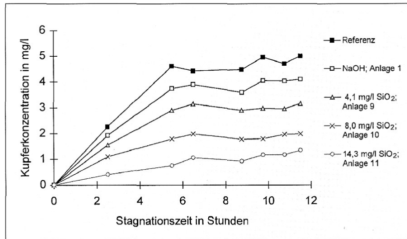
Abb. 3: Kupferkonzentration des Wassers in Abhängigkeit der Stagnationszeit in Kupferrohren; Alter der Deckschicht: 200 Tage (2)
